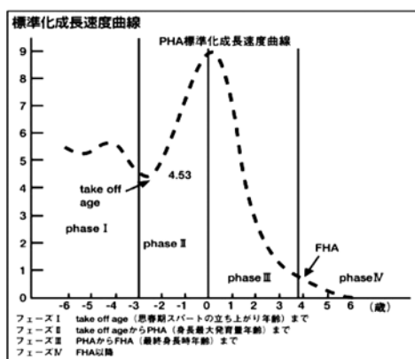
図1 標準化成長速度曲線
